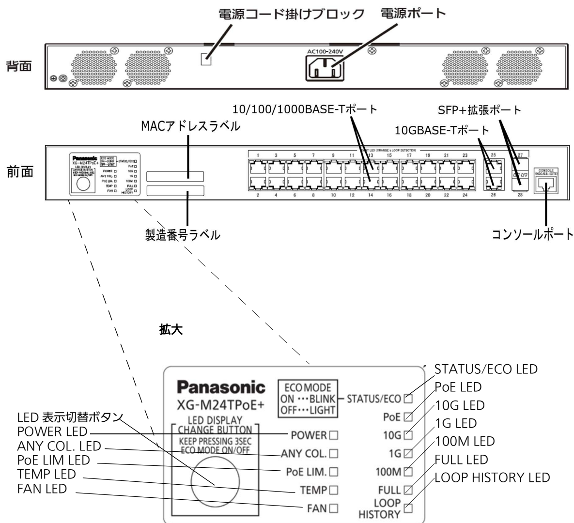
図 1-1 XG-M24TPoE+ 外観図
