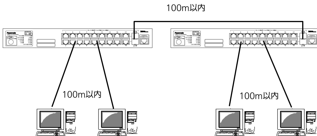
図3-1 接続構成例
