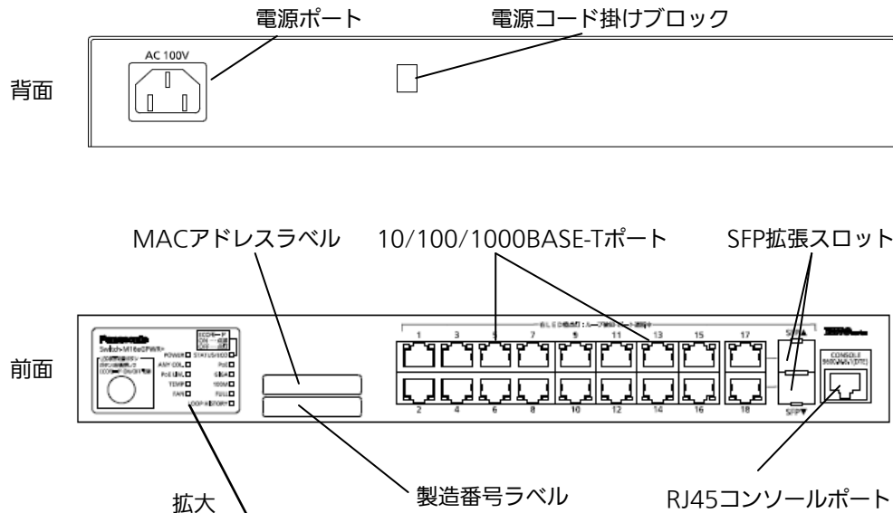
図 1-1 Switch-M16eGPWR+
