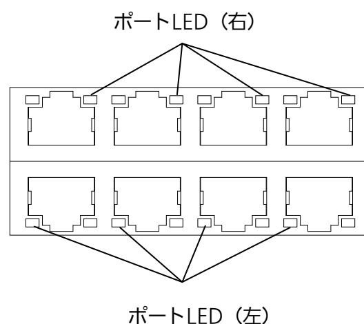
図 1-5 ポート LED
