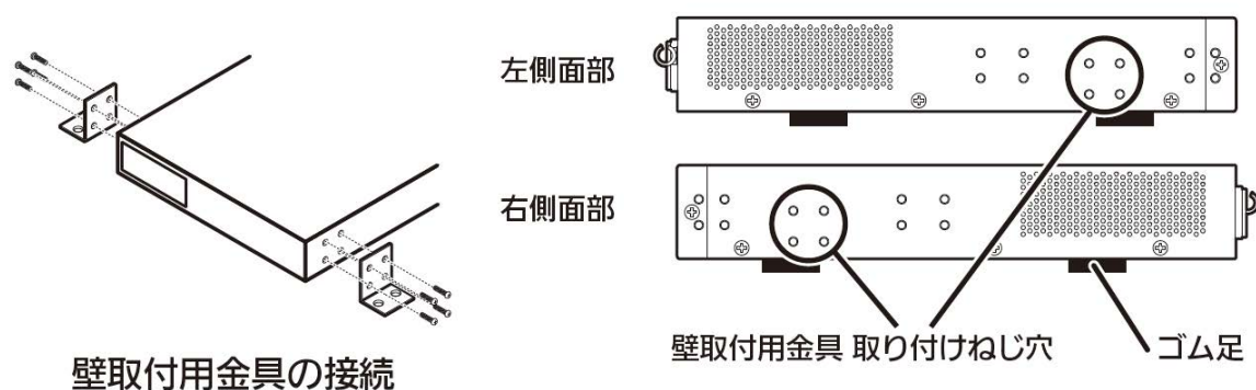
図 2-3 壁面への設置
