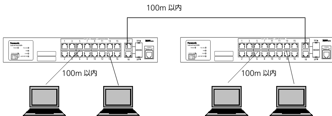
図 3-1 接続構成例
