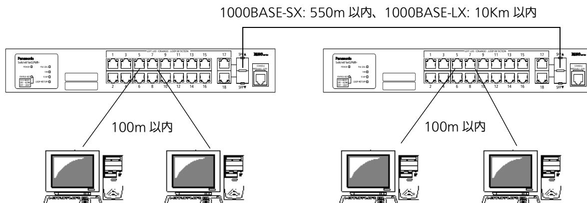
図 3-2 光ファイバケーブル接続例
