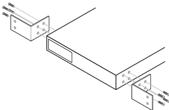
図 2-2 ラックへの設置
