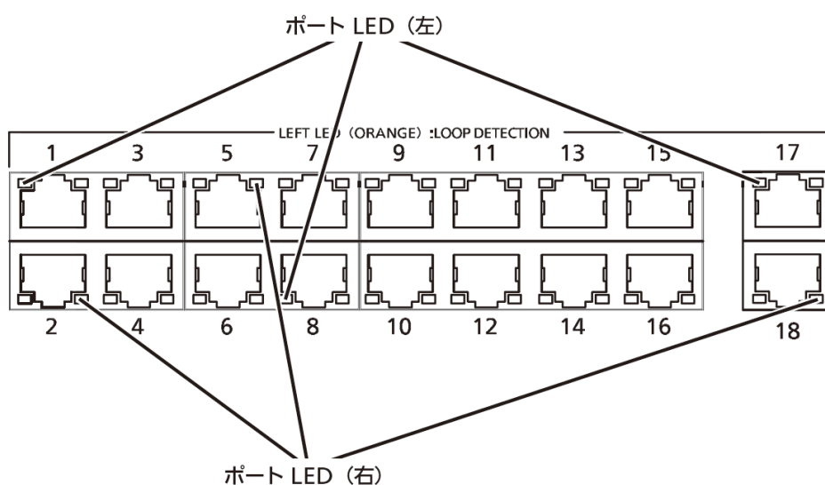
図 1-2 ポート LED
