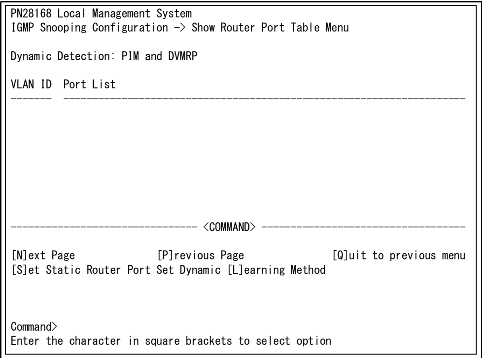
図 4-6-8-4 ルータポートテーブル参照
