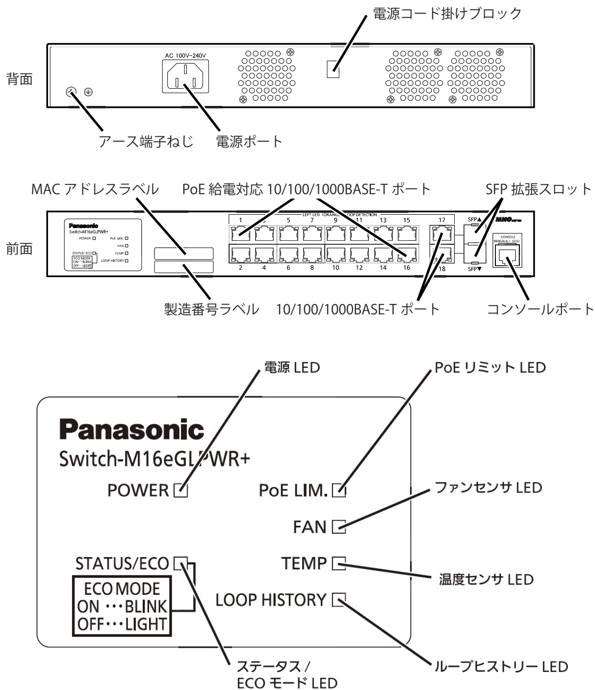
図 1-1 各部の名称
