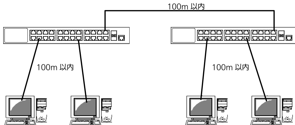
図 3-2 接続構成例
