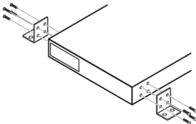
図2-2 壁面への設置
