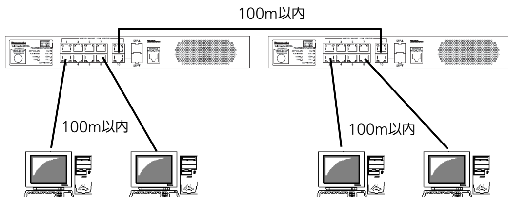
図3-1 接続構成例
