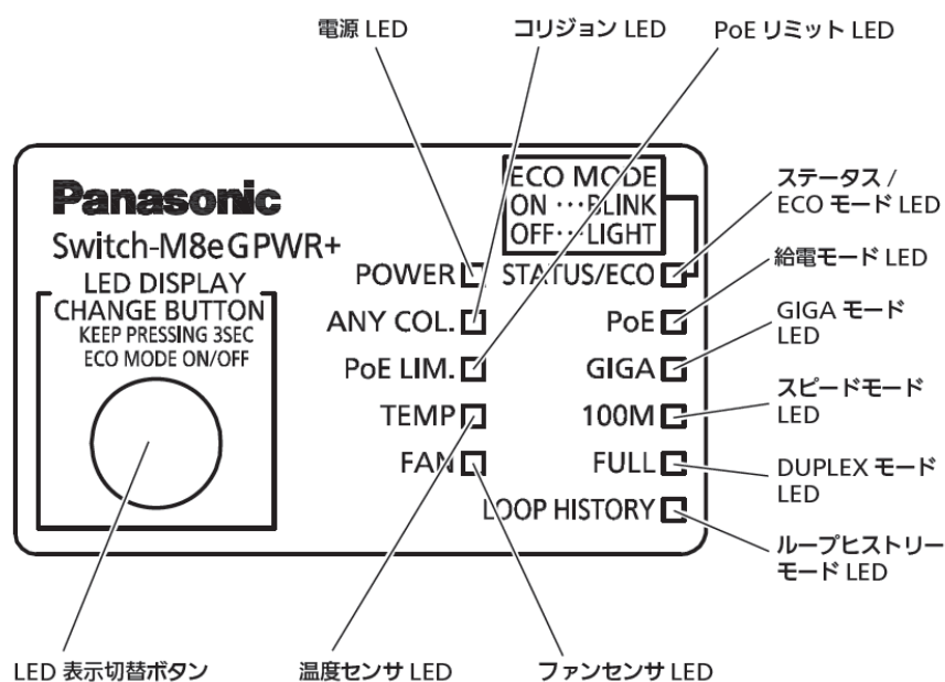
図1-2 前面LED拡大図
