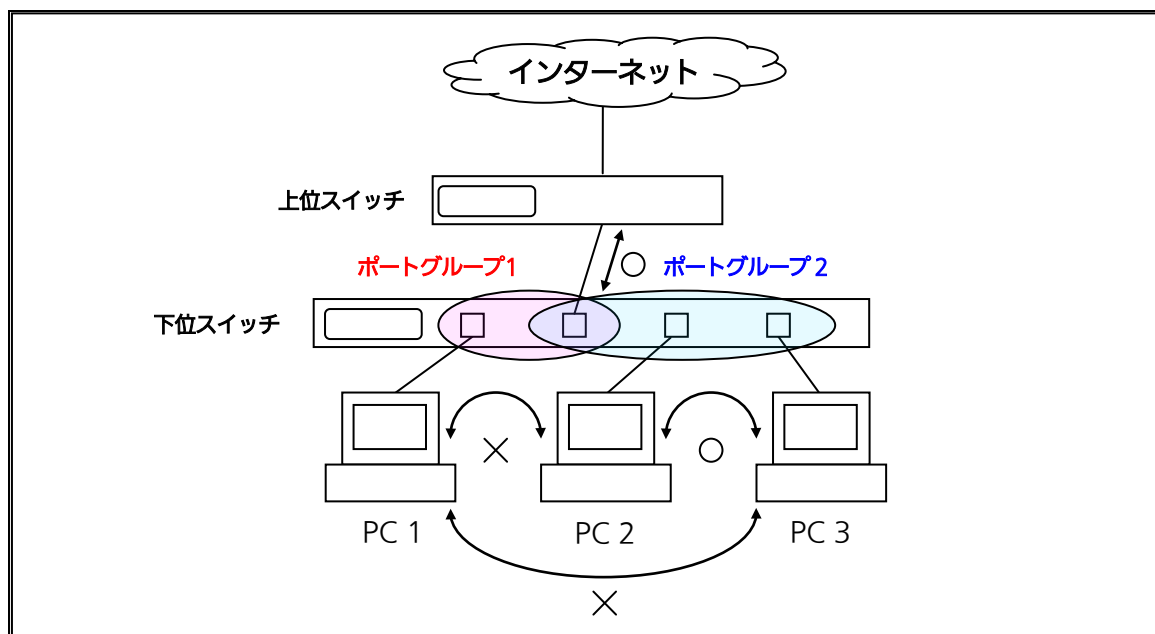
図4-7-56 ポートグループピングを利用した構成例 (PC1ーインターネット間、PC2ーPC3ーインターネット間を通信可能とさせる構成)
