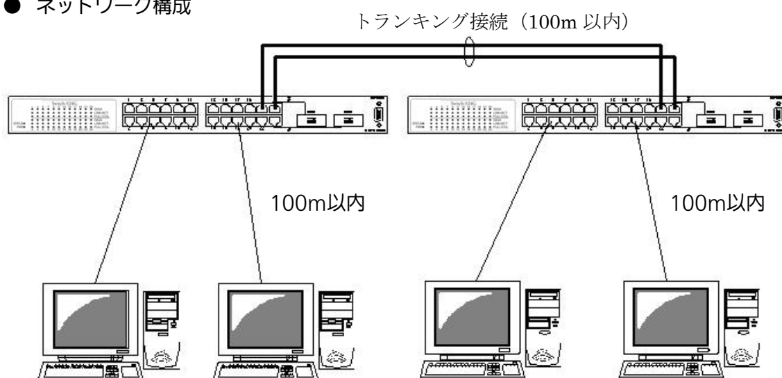
図3-1 接続構成例
