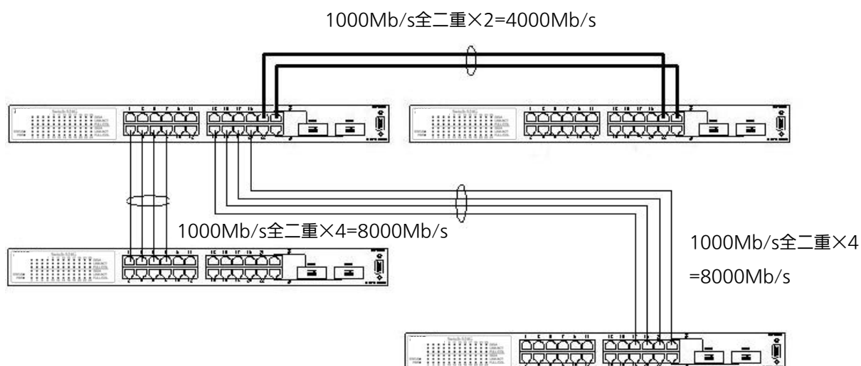
図4-7-7 トランキングを用いた構成例 2
