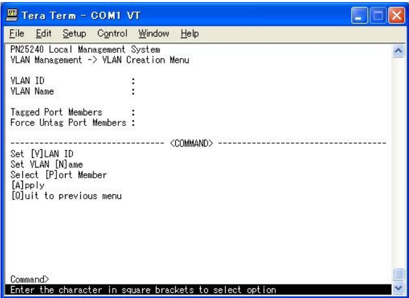
図4-7-3 VLANの作成
