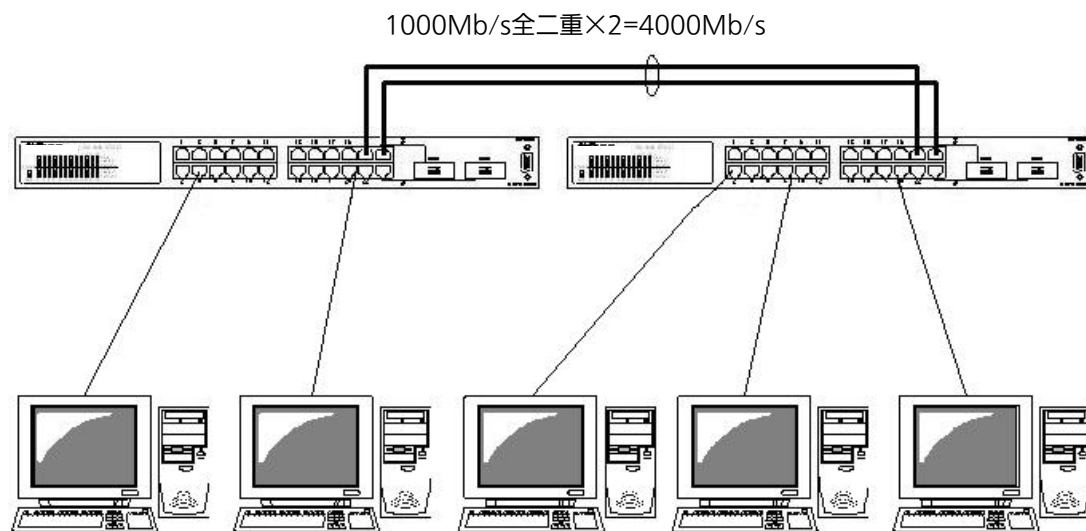
図4-7-6 トランキングを用いた構成例 1
