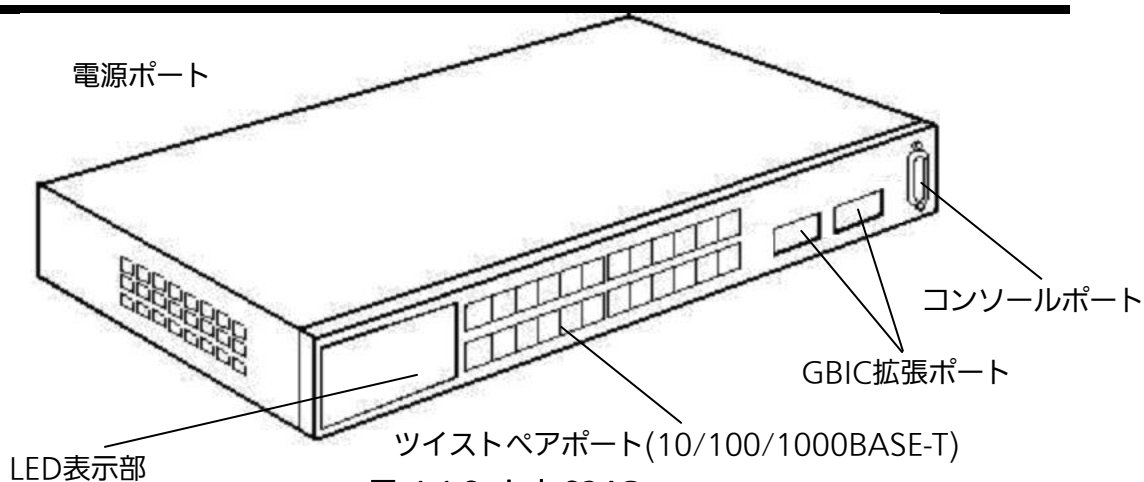
図 1-1 Switch-S24G
