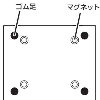
Switch-M16PWR 底面部
