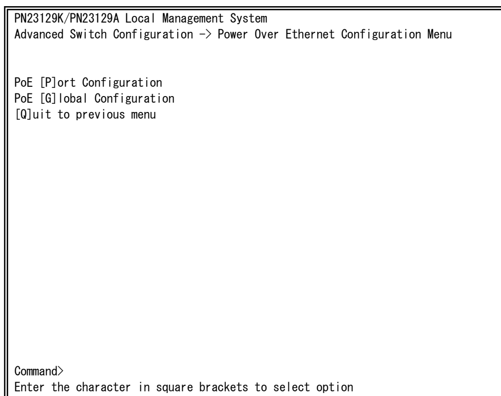
図4-7-51 PoEの設定
