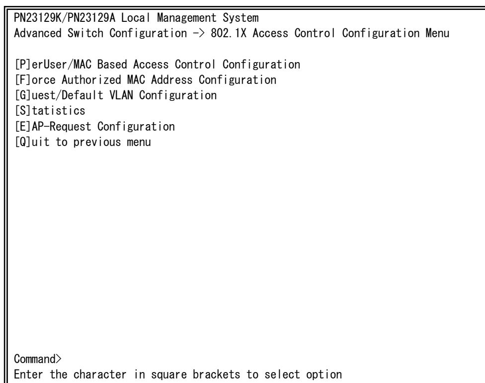
図4-7-36 IEEE802.1x認証機能
