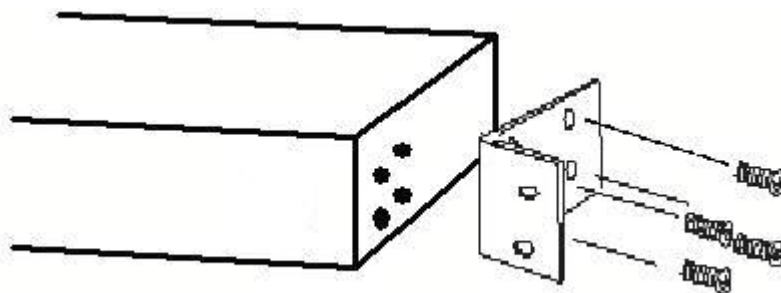
図2-1 19インチラックへの設置
