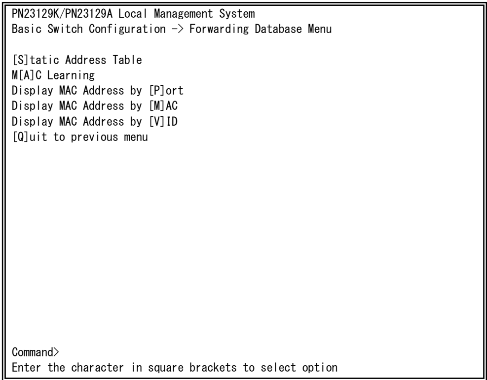
図4-6-16 MACアドレステーブルの参照
