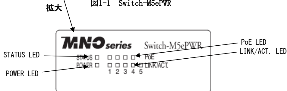
図1-2 前面LED拡大図
