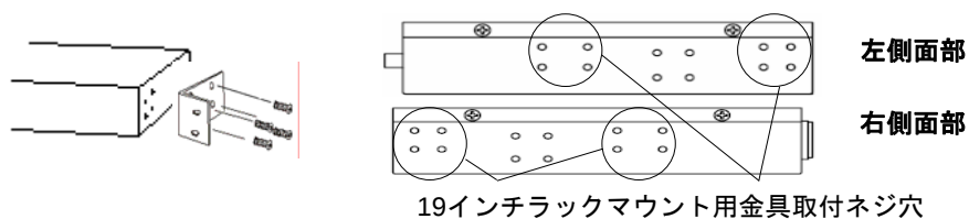
図2-2 19インチラックマウント用金具位置
