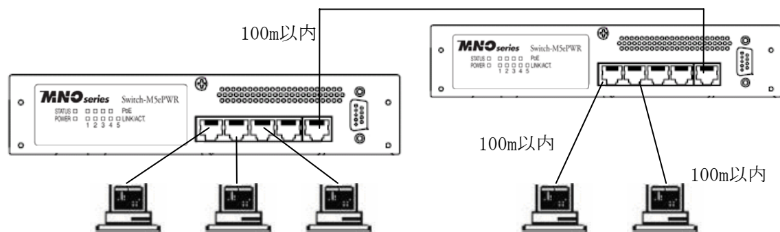
図3-1 接続構成例
