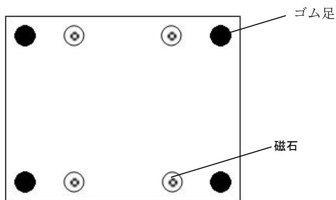
図2-1 スチール面への取り付け
