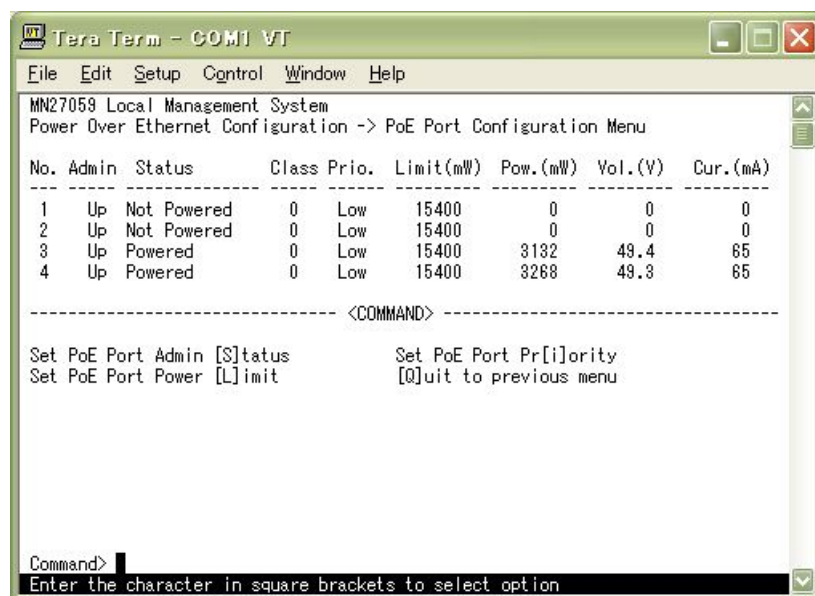
図4-7-8 各ポートの設定
