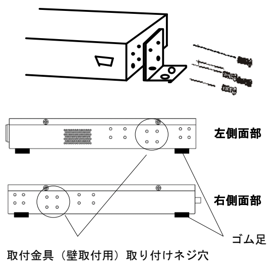
図2-4 壁面への取り付け
