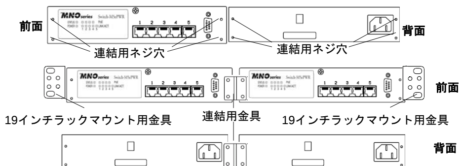
図2-4 19インチラックへの設置（2台連結の場合）
