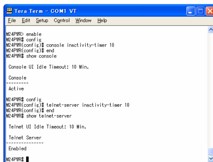
図 3-7 Console(show console)、Telnet server (show telnet-server)の設定情報参照
