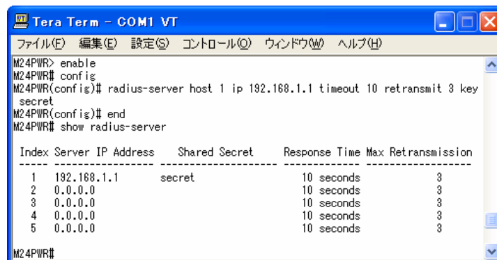
図 3-9 RADIUS サーバ の設定参照(show radius-server)
