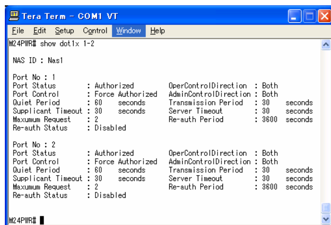
図 4-10 IEEE802.1x 認証設定参照 (show dot1x 1-2)
