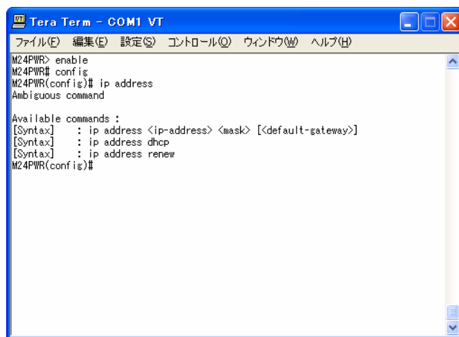
図 1-4 候補支援コマンド
