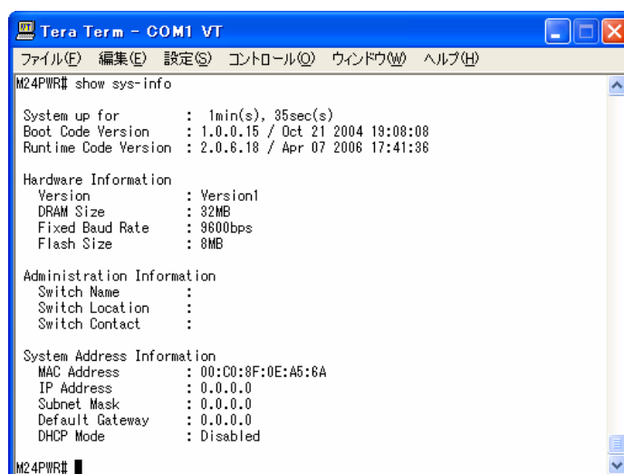
図 2-1 基本情報参照 (show sys-info)
