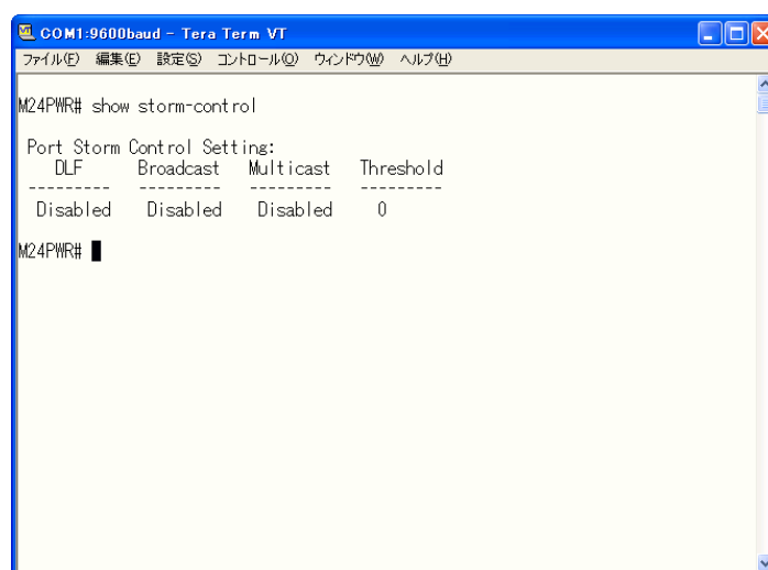
図 4-14 ストームコントロール設定参照 (show storm-control)
